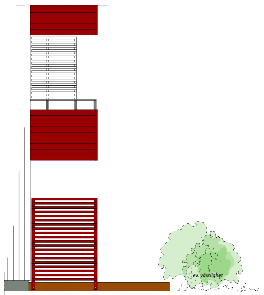
ELEVATION, alternativ A och C
