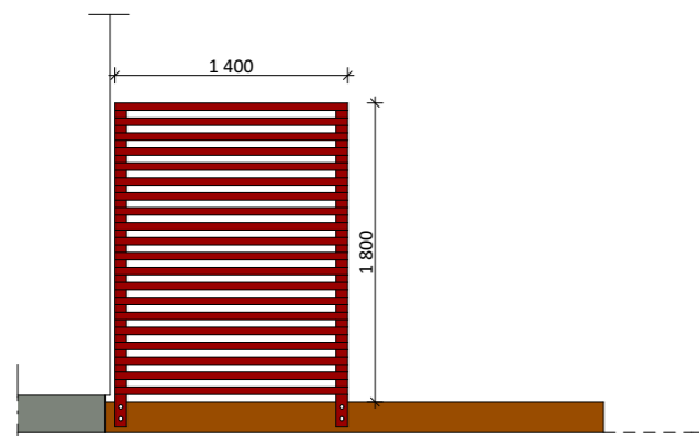
Altan alternativ A Elevation
