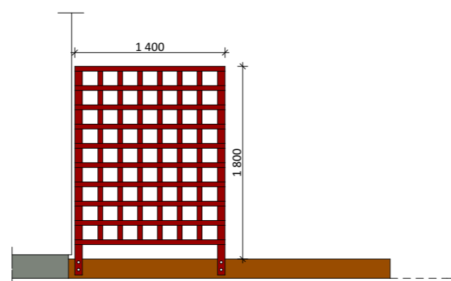
Altan alternativ B Elevation
